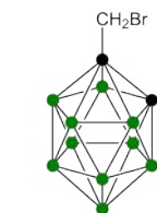
1-(CH 2 Br)-1,2-C 2 B 10 H 11
