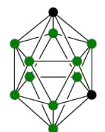
1,7-C 2 10 B 10 H 12
