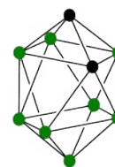
1,2-C 2 B 8 H 10
