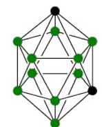
1,7-C 2 11 B 10 H 12
