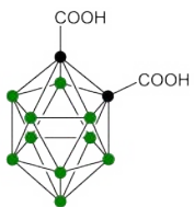
1,2-(CO 2 H) 2 -1,2-C 2 B 10 H 10
