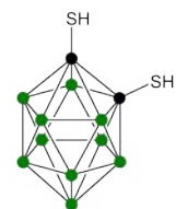
1,2-(SH) 2 -1,2-C 2 B 10 H 10
